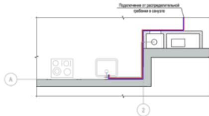
Фрагмент плана в осях А/2 с разводкой систем Т3, В1, К1
